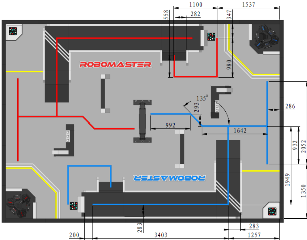
图 3-3 场地引导线
